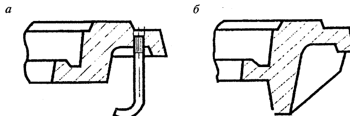
Рисунок А.4 — Усиленная заделка корпуса люка
