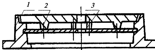
Рисунок А.2 — Люк, оснащенный запорным замковым устройством
